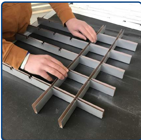
Inserire listelli Tipo A Maschio Insert the blade Type A Male
