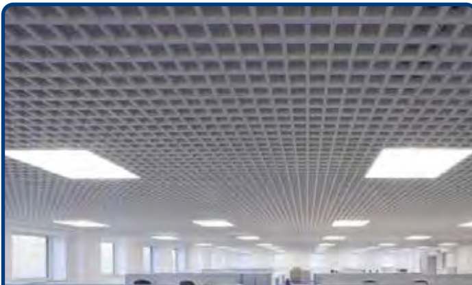
GRIGLIATI CARABOTTINO Grigliati schermanti passanti maglia quadrata e rettangolare. Ispezionabili in appoggio su struttura T e continuità visiva senza interruzione. Alluminio preverniciato.
