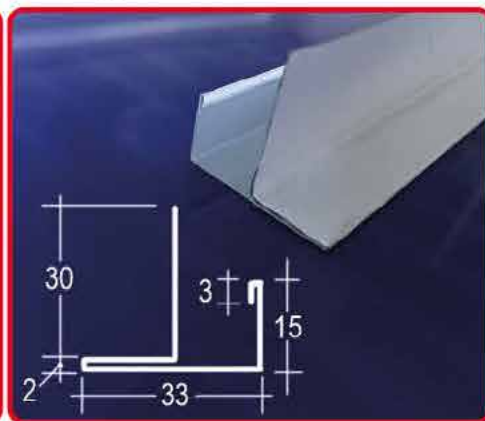
Type RU 13mm - 16mm
